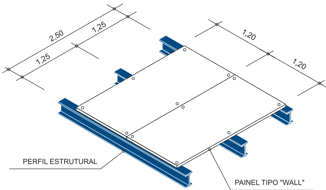
Fig. 1 - Disposição e fixação recomendada para instalação correta do painel tipo "wall"
