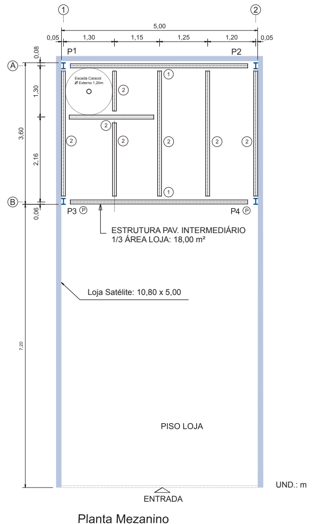
Figura 3.a - Dimensões do mezanino para loja satélite de 54 m 2
